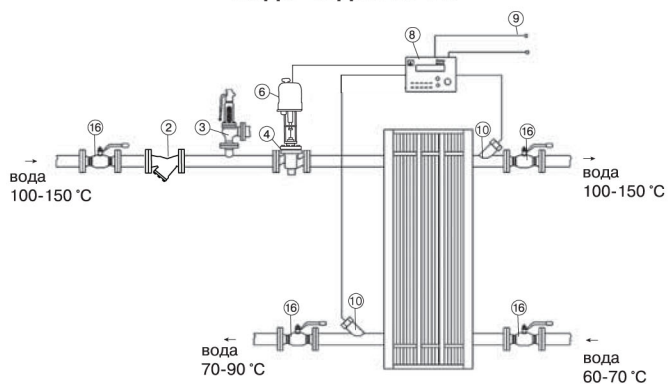
Водо-водяные ТО
