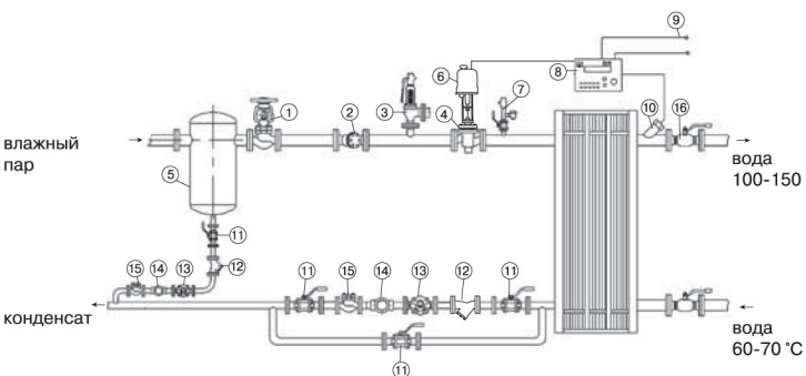
Пароводяные ТО
